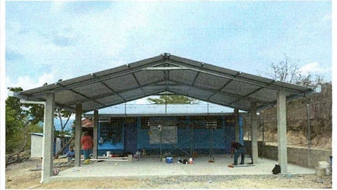
Foto 2: MEJORAMIENTO CON ESTRUCTURA TIPO PÓRTICO E INSTALACIÓN DE LÁMINAS TROQUELADA CALIBRE 26, PARA AREA DE REUNIONES FINALIZADO.
